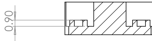
SECTION A-A SCALE 3 : 1
